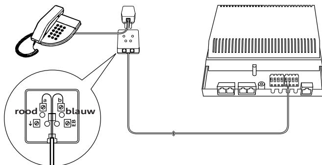
Afbeelding 4: Apparatuur via een telefoonstopcontact aansluiten op de Quattrovox
