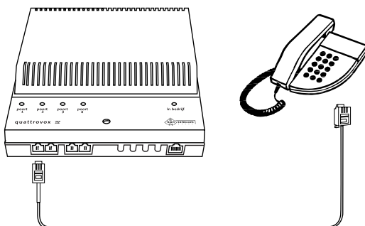
Afbeelding 3: Analoge telefoon aansluiten op de Quattrovox.
